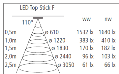
Curva de distribución luminosa
