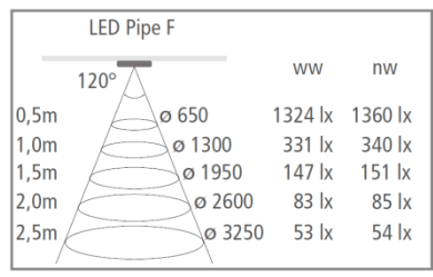
Curva de distribución luminosa
